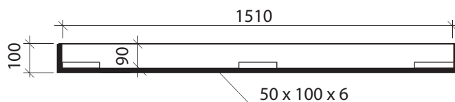
Leikkaus
