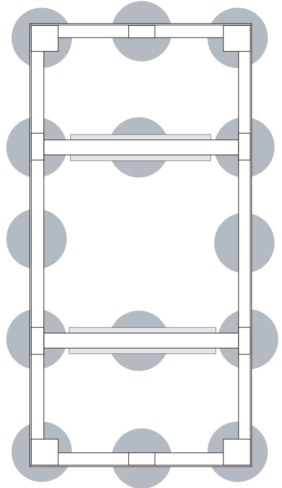
Asennuskehikko 1500 x 3000
